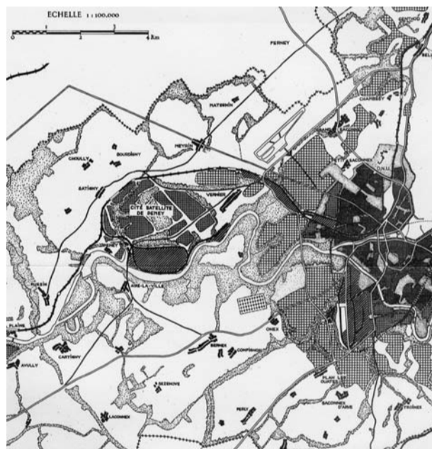
LA CITÉ SATELLITE DE PENEY. PLAN DIRECTEUR DU DÉPARTEMENT DES TRAVAUX PUBLICS, 1945. ARCHIVES TETU-HEPIA
